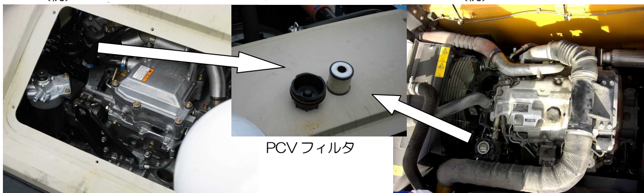
(例) KR-25H-V7
