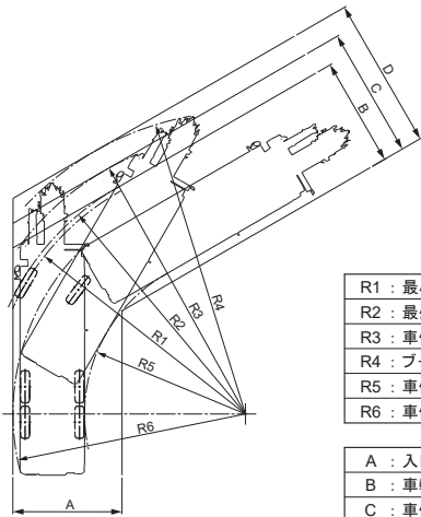
2輪ステアリングで右折する場合
